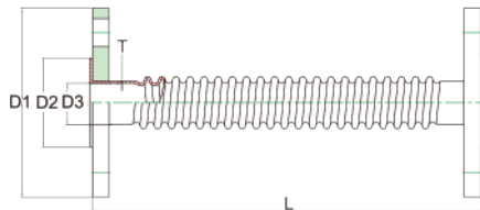
法蘭：ANSI Class 150
