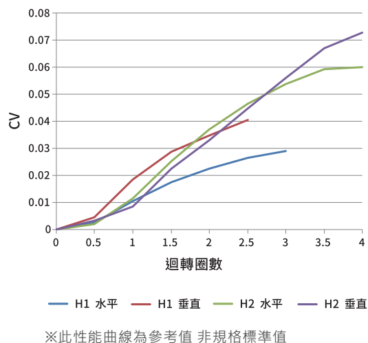
CV值性能曲線
