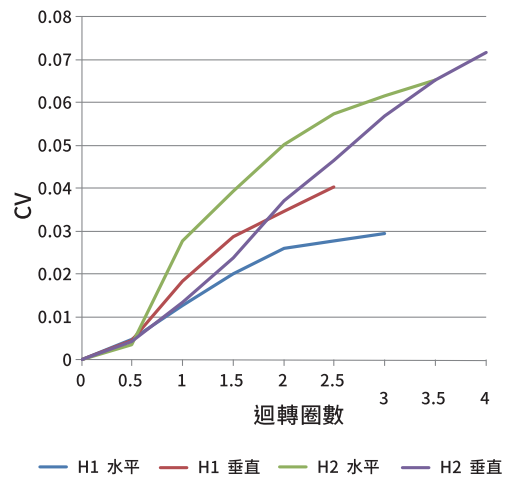
CV值性能曲線
